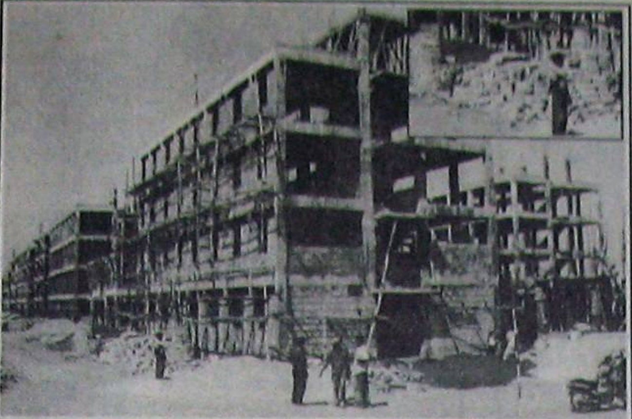
రాజీవ్ గృహకల్ప పథకంలో భాగంగా నెల్లూరు ఇరుగాళమ్మ గుడి వద్ద నిర్మితమవుతున్న అపార్ట్ మెంట్. బూడిద సిమెంట్ తో తయారు చేసిన ఇటుకలు దీనికి వినియోగిస్తున్న వైనాన్ని ఇన్ సెట్ లో చూడొచ్చు.
